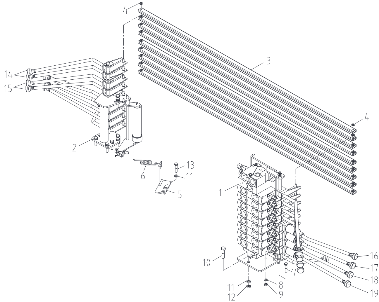
오퍼레이션 메인 조립체 Fig. 3-4 SCS514 OPERATION MAIN ASS'Y
