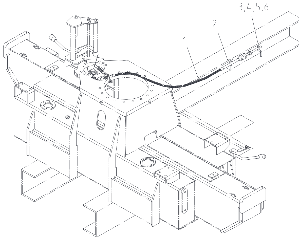
악셀 시스템 파트 Fig. 8-3 SCS514 ACC' SYSTEM PART
