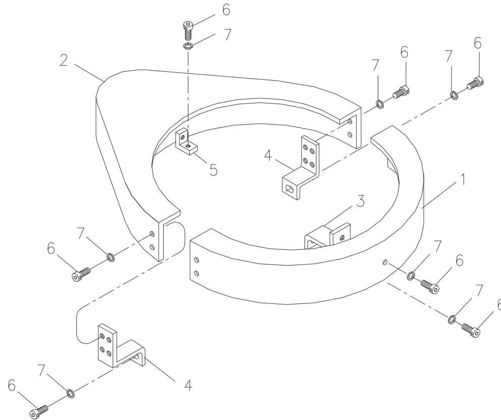
스윙 커버 조립체 Fig. 3-5 SCS514 SWING COVER ASS'Y
