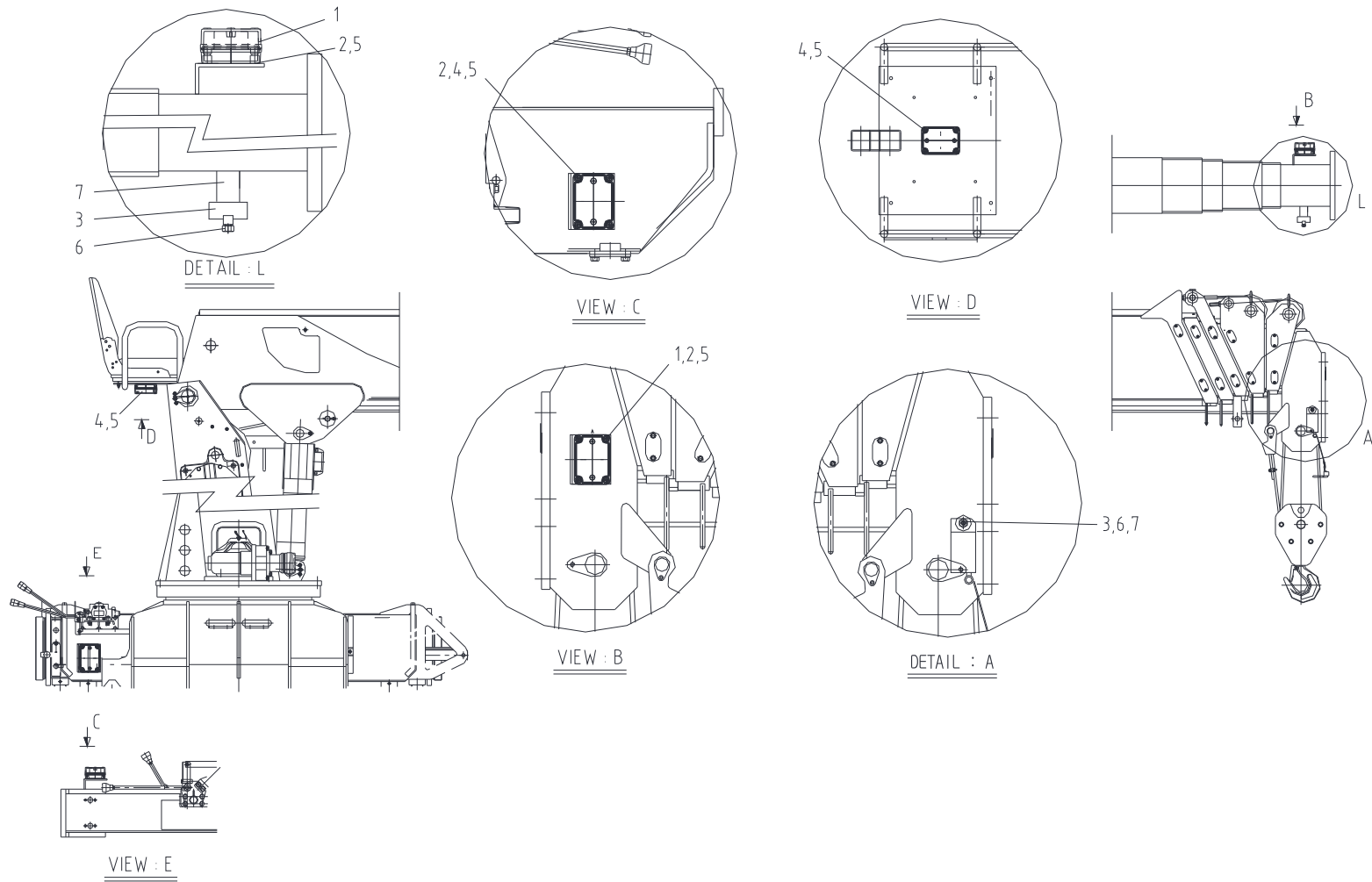
무선 과권 장치 위치도 Fig. 9-3-1 SCS514 BOOM WIRING
