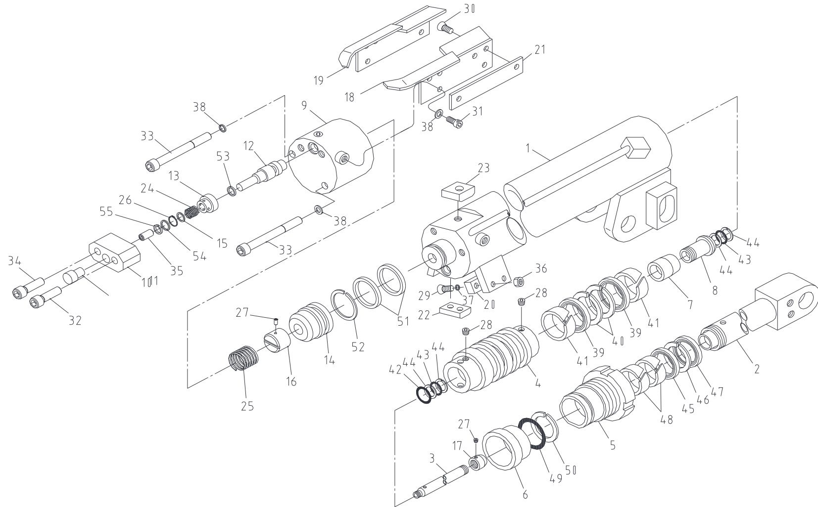
텔레스코픽 실린더 1단 조립체 Fig. 1-1-1 SCS514 TELESCOPIC CYL'(1st) ASS'Y
