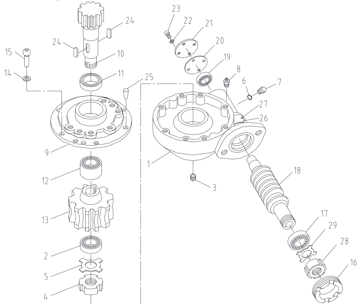
스윙 감속기 세트 Fig. 3-1 SCS514 SWING R/G SET
