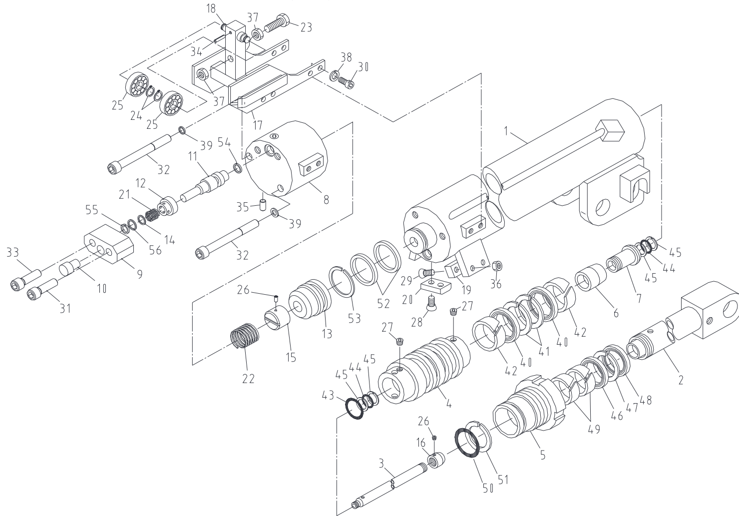
텔레스코픽 실린더 (2단) 조립체 Fig. 1-1-2 SCS514 TELESCOPIC CYL (2nd) ASS'Y
