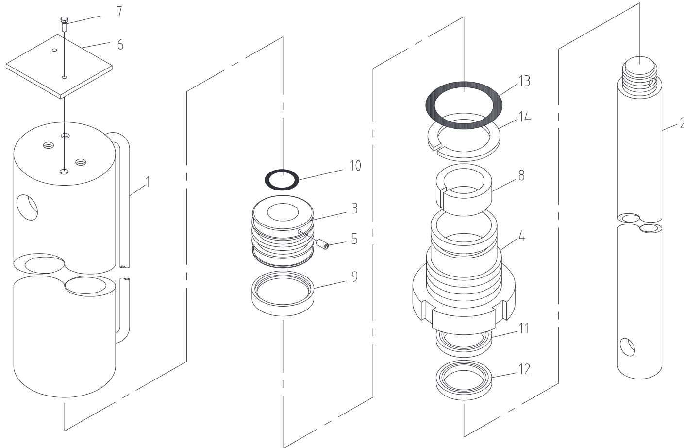
잭 실린더 조립체 Fig. 4-1 SCS514 JACK CYL' ASS'Y
