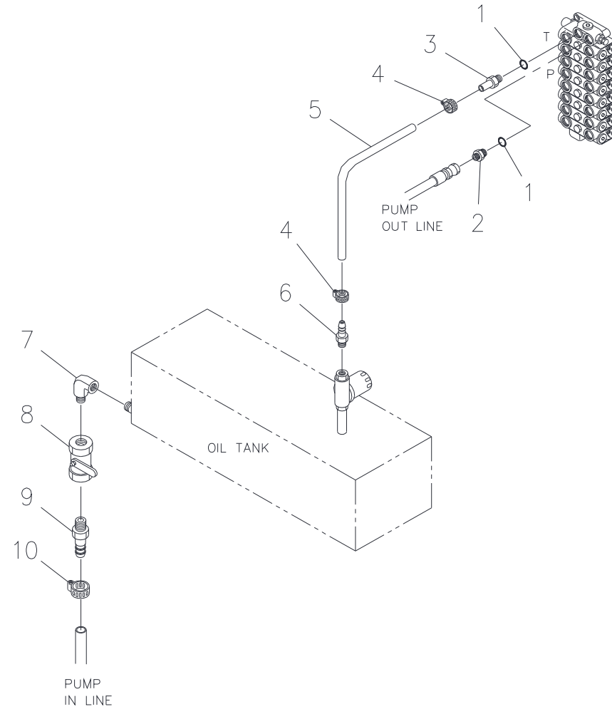
디스트리뷰터 배관 Fig. 5-1 SCS514 DISTRIBUTOR PIPING
