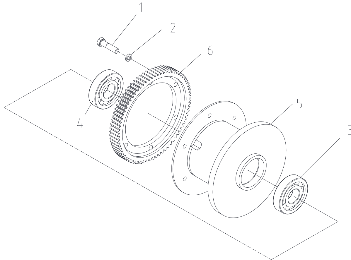
드럼 조립체 Fig. 2-1 SCS514 DRUM ASS'Y
