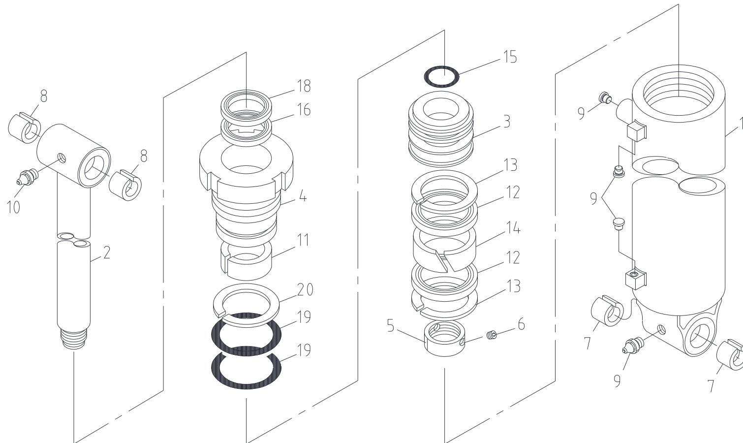
데릭 실린더 조립체 Fig. 2-3 SCS514 DERRICK CYLINDER ASS'Y
