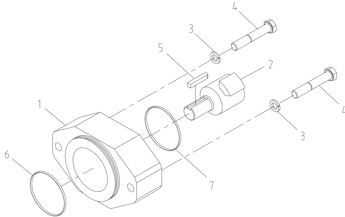
스윙 감속기 아답터 조립체 Fig. 3-2 SCS514 SWING R/G ADAPTER ASS'Y
